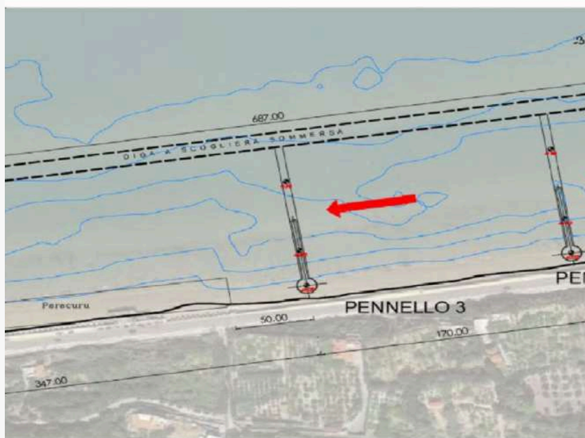
Figura 9. Area di intervento – Pennelli dal nr. 2 al nr. 5
